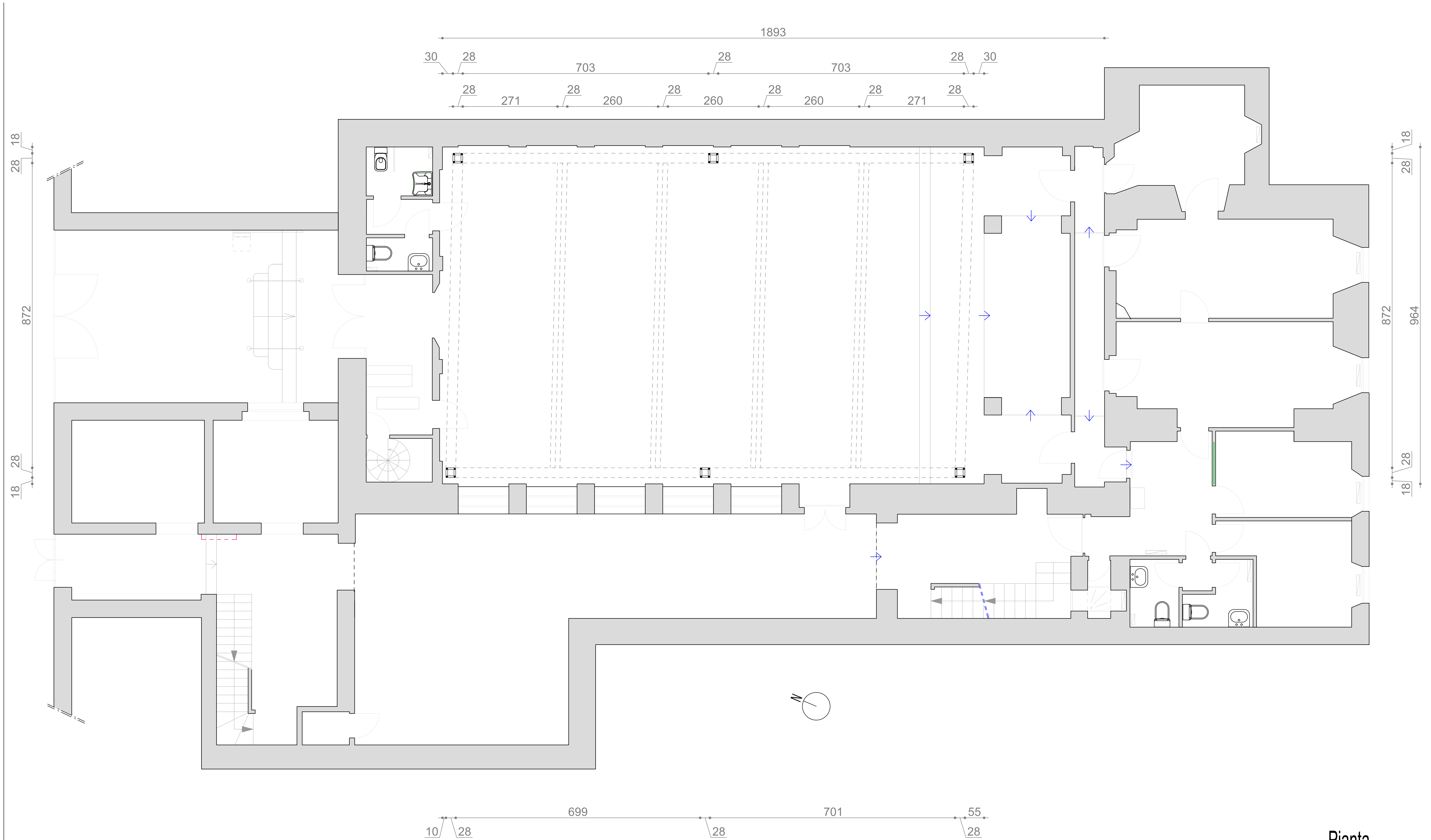
Pianta
